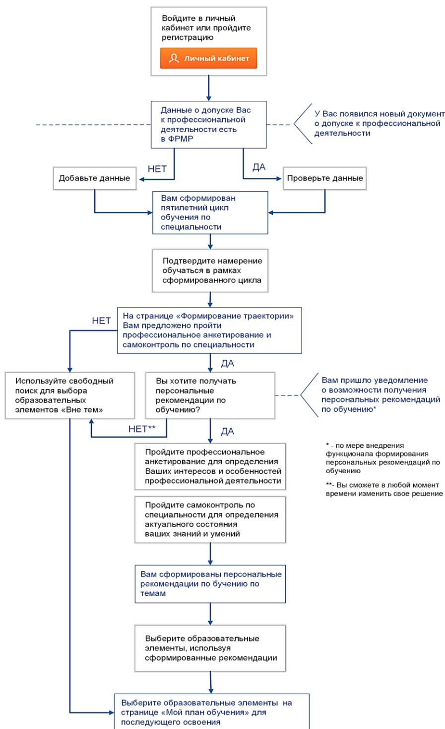
Схема 7. Алгоритм работы на Портале
